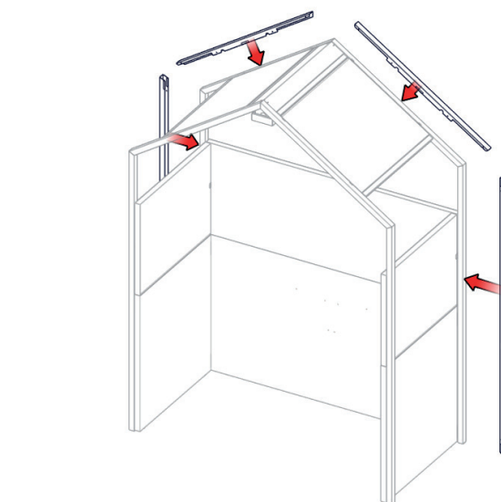
plaatsing optionele kabelafdekking in contour van huisje
