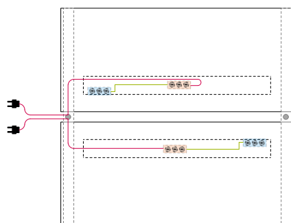
bovenaanzicht duo-werkplek
